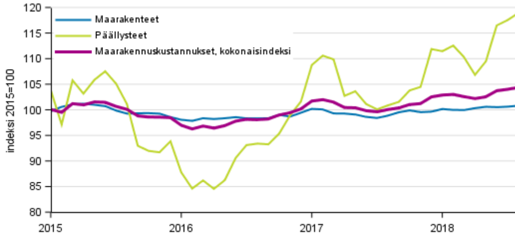
Liitekuvio 1. Maarakennusindeksin (2015=100) kokonaisindeksin, maarakennetöiden ja päällysteiden kustannuskehitys 1/2015–8/2018
